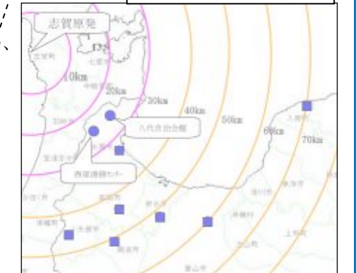
モニタリングポスト配置図
