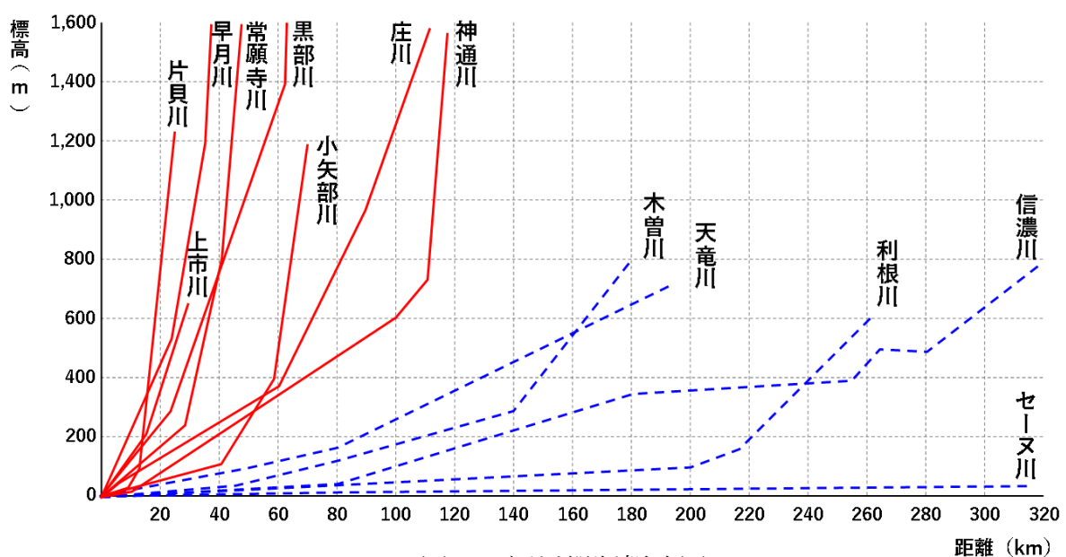
図4 河川縦断概略図
