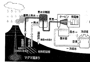
地熱発電のしくみ
