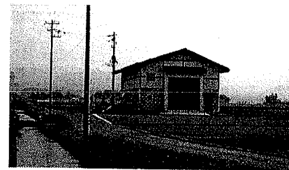
農業用水を活用した 仁右門用水発電所
