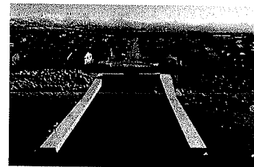
河川(放水路)の整備(沖田川放水路)
