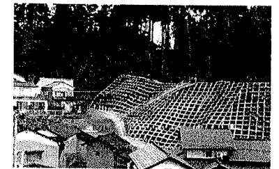
急傾斜地崩壊防止施設の整備(水見市朝日丘地区)
