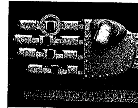
ロボットハンド用超薄型フレキシブル触覚センサ
