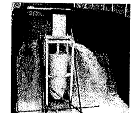
低落差(1m)でも効率的な発電可能なマイクロ水力発電機
