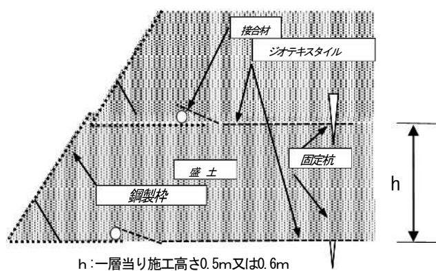
図① 鋼製杭タイプ施工数量標準図
