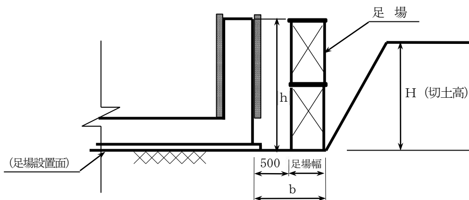
図 2-7 足場設置の場合<参考図>
