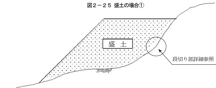
図2-25 盛土の場合①
