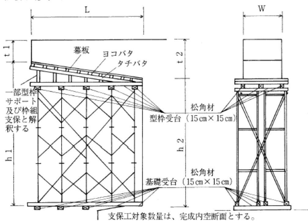
支保工概念图（参考例）
