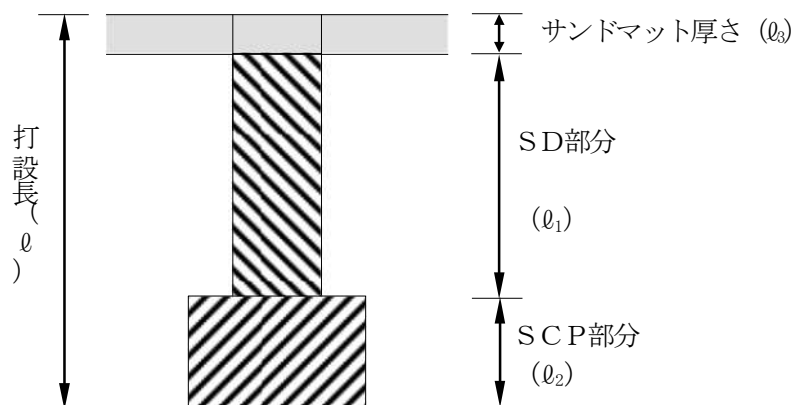
図ー2 サンドドレーン・サンドコンパクションパイル併用工
