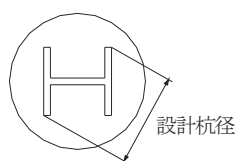
H形鋼の場合
