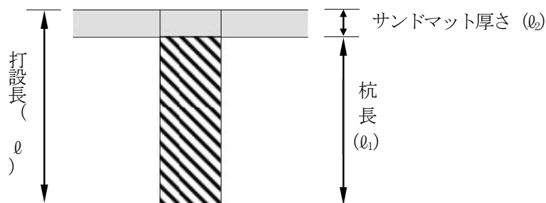
図ー1 サンドドレーン及びサンドコンパクションパイル
