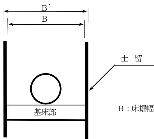
図２－４ 土留施工の床掘幅（砂・碎石基礎）
