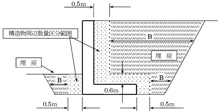
図2-32 擁壁の場合
