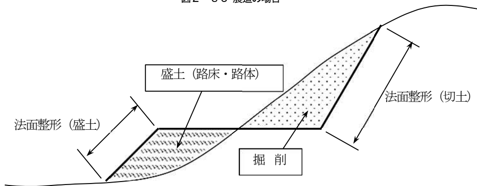
図2-35 農道の場合
