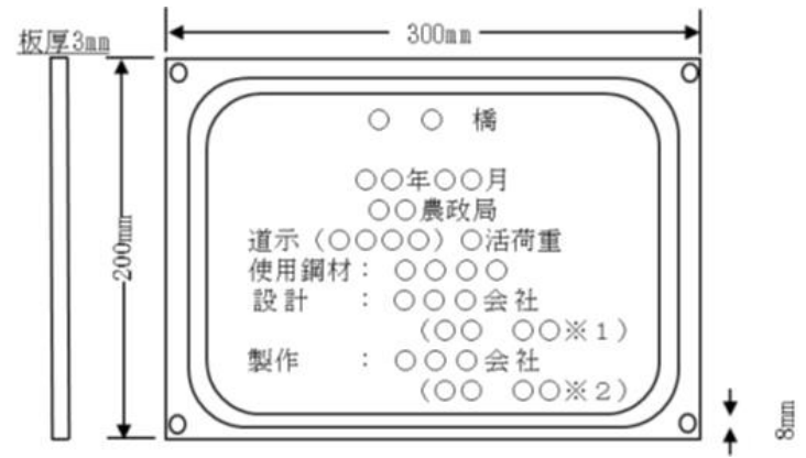
※ 1 管理技術者氏名、※ 2 監理技術者氏名 図 10－ 1 － 1 銘板の寸法及び記載事項
