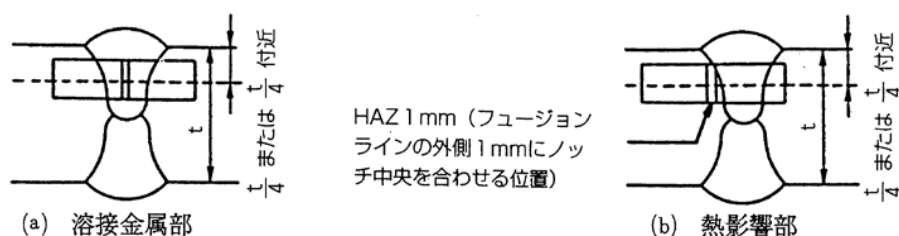
圖 3-3-2 衝擊試驗片採取位置
