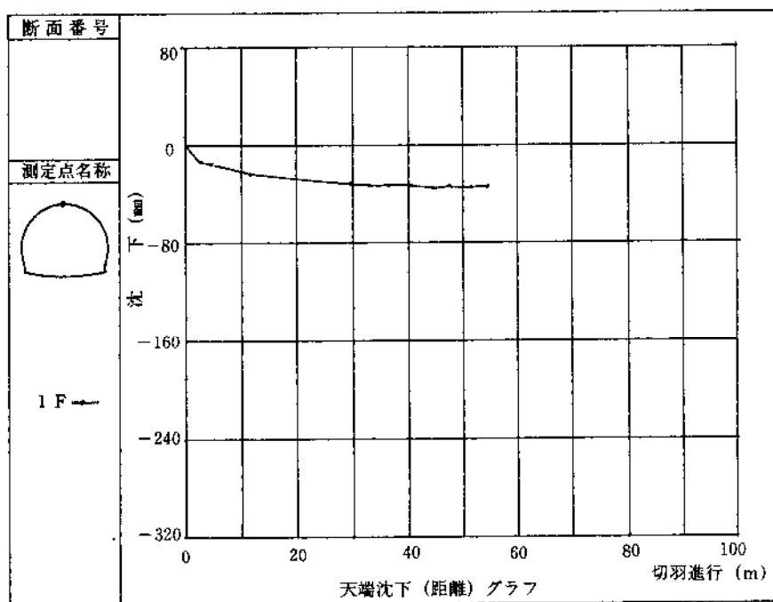
図－４ 天端沈下変化図(例)
