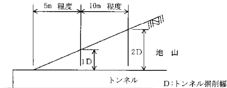
図－9 地表沈下の測定間隔
