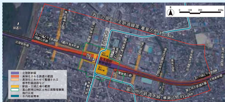
富山駅付近連続立体交差事業 概要図
