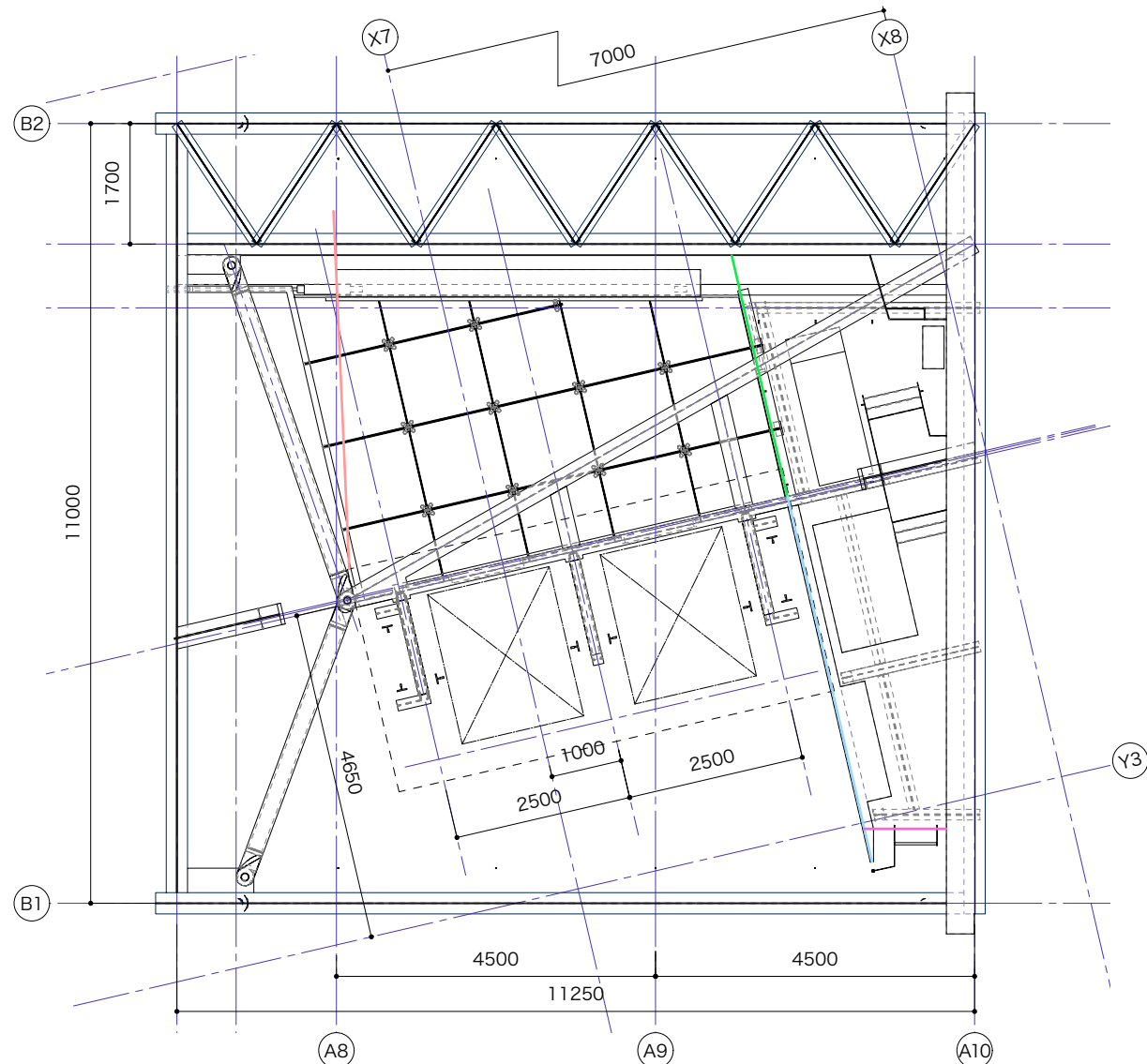
7FL+3734.5 平面図 S=1/100(A3)
