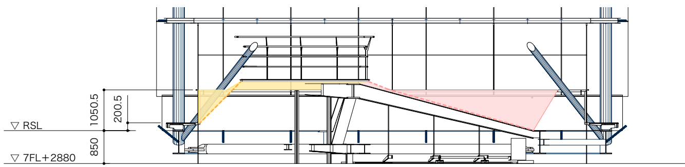
C 断面図 S=1/100(A3)
