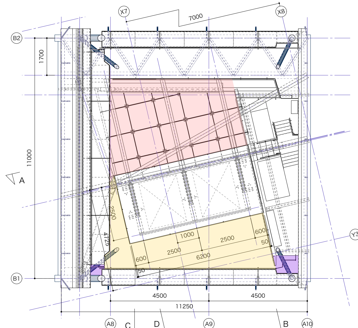
EV機械室 平面図 S=1/100(A3)
