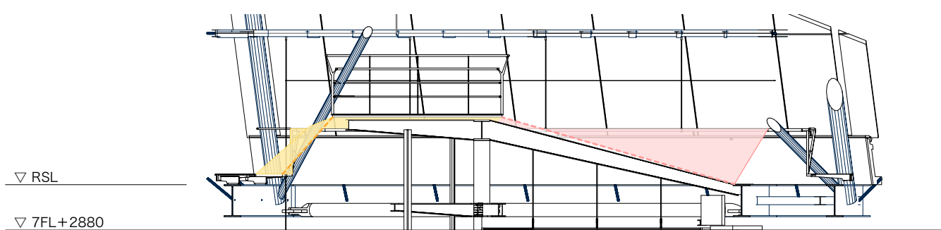
D 断面図 S=1/100(A3)
