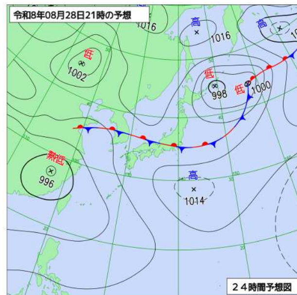
8月28日21時の予想天気図
