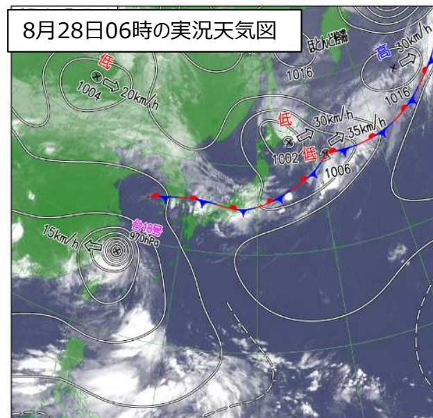
気象衛星ひまわり（赤外画像）を重ねた天気図
