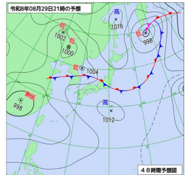
8月29日21時の予想天気図
