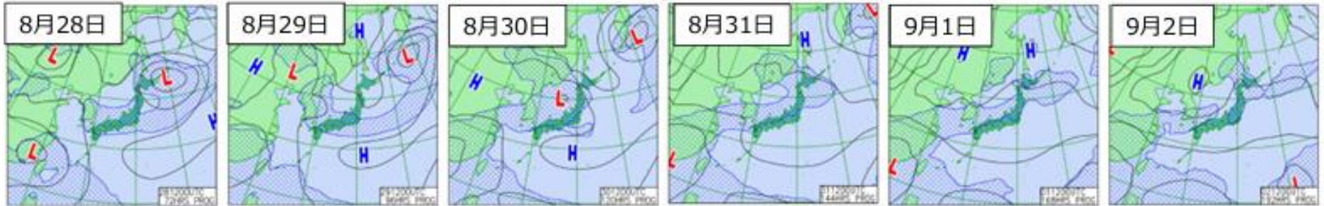
上図のHは高気圧、Lは低気圧、ハッチ掛けのある部分は、24時間に5ミリ以上の降水が予想されている領域を示しています。
