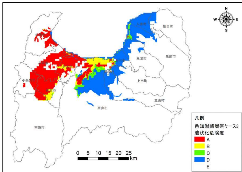
図5.8 邑知潟断層帯ケース3の地震による液状化危険度
