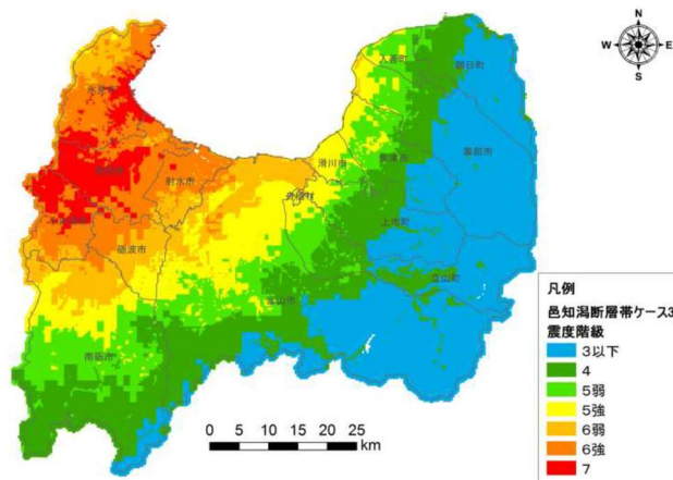
図 4. 8 邑知潟断層帯ケース 3 地震予想震度分布
