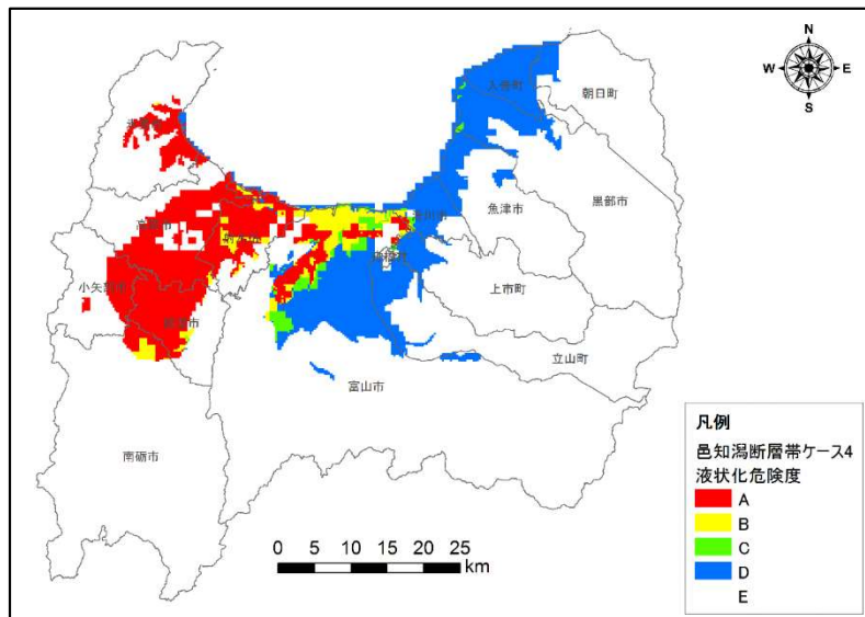
図5.9 邑知潟断層帯ケース4の地震による液状化危険度
