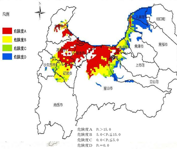
図 5.2 呉羽山断層地震液状化判定結果図
