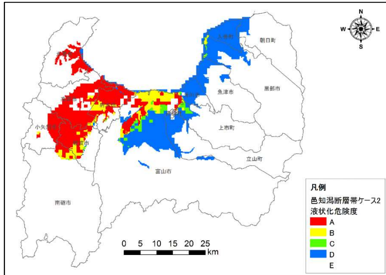
図5.7 邑知潟断層帯ケース2の地震による液状化危険度
