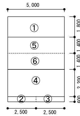
図5 1階平面図 1/500
