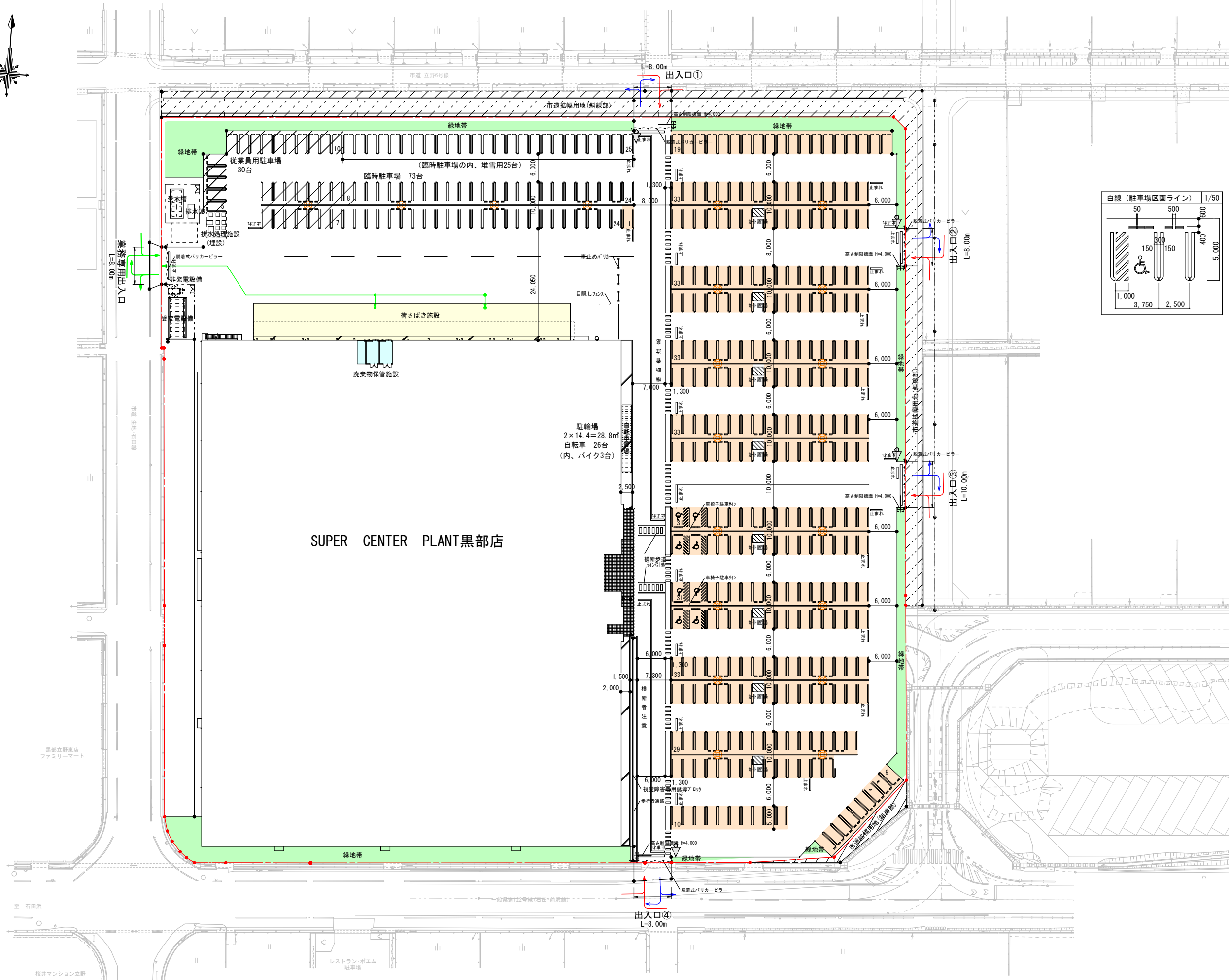
図3 建物配置図（変更前） 1/800
