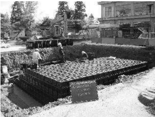
立山町 雨水貯留浸透施設の整備 (立山町役場駐車場)
