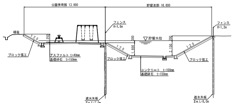
貯留池本体工 標準断面図
