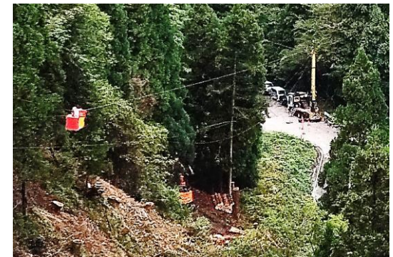
タワーヤードによる効率的な集材
