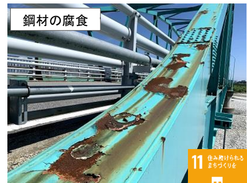
県道魚津生地入善線 下黒部橋の老朽化対策
