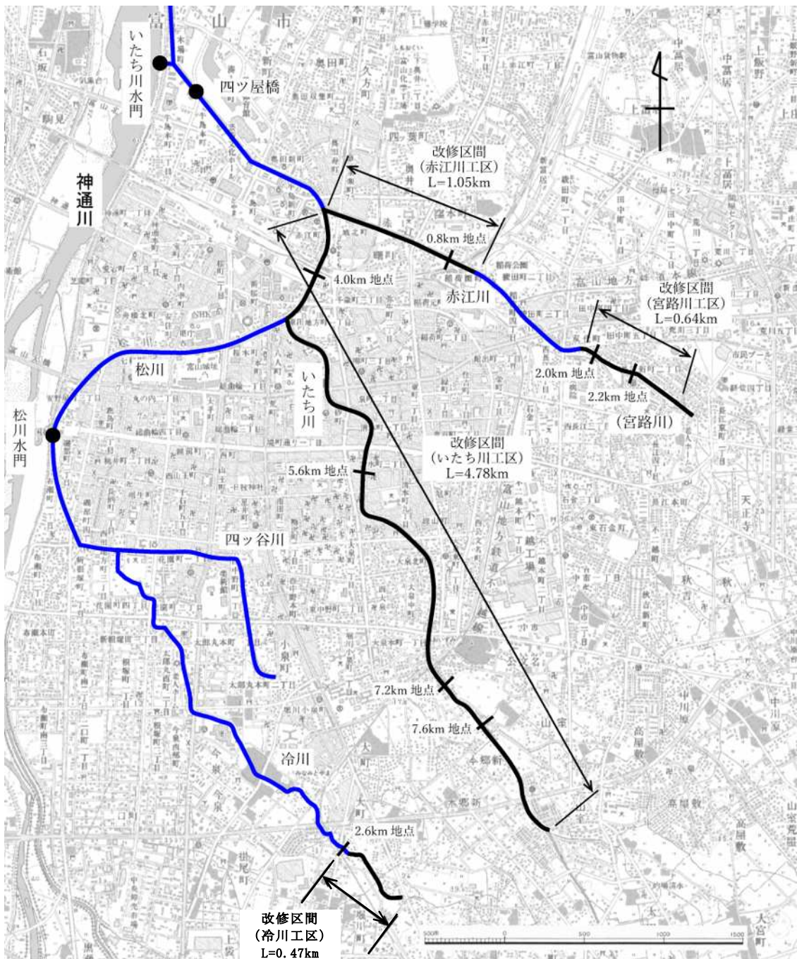
図3-1 施行区間位置図
