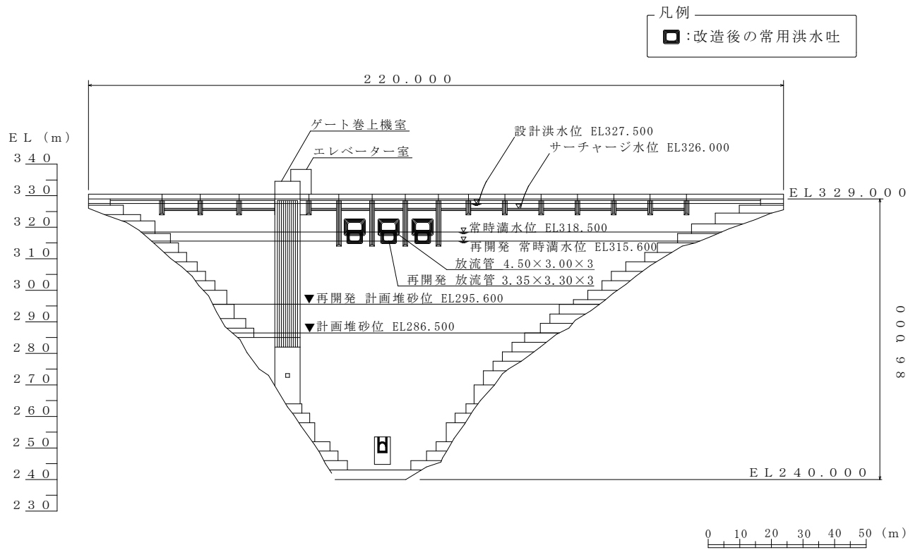
図 3 - 1 1 上流面図
