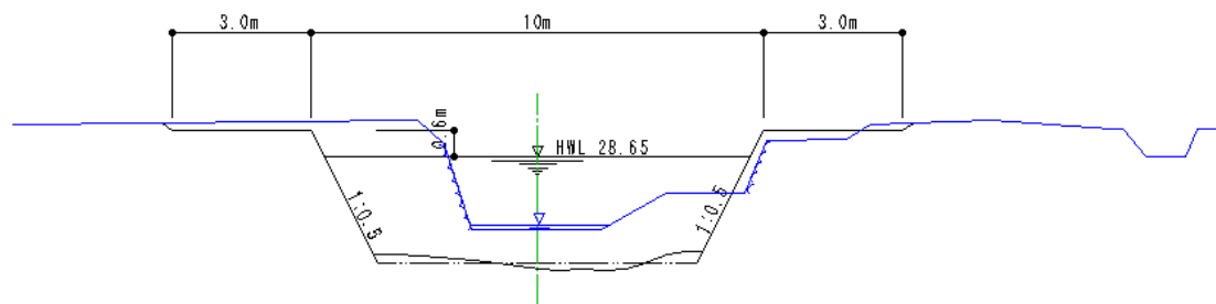
図 3 - 6 標準横断面図
