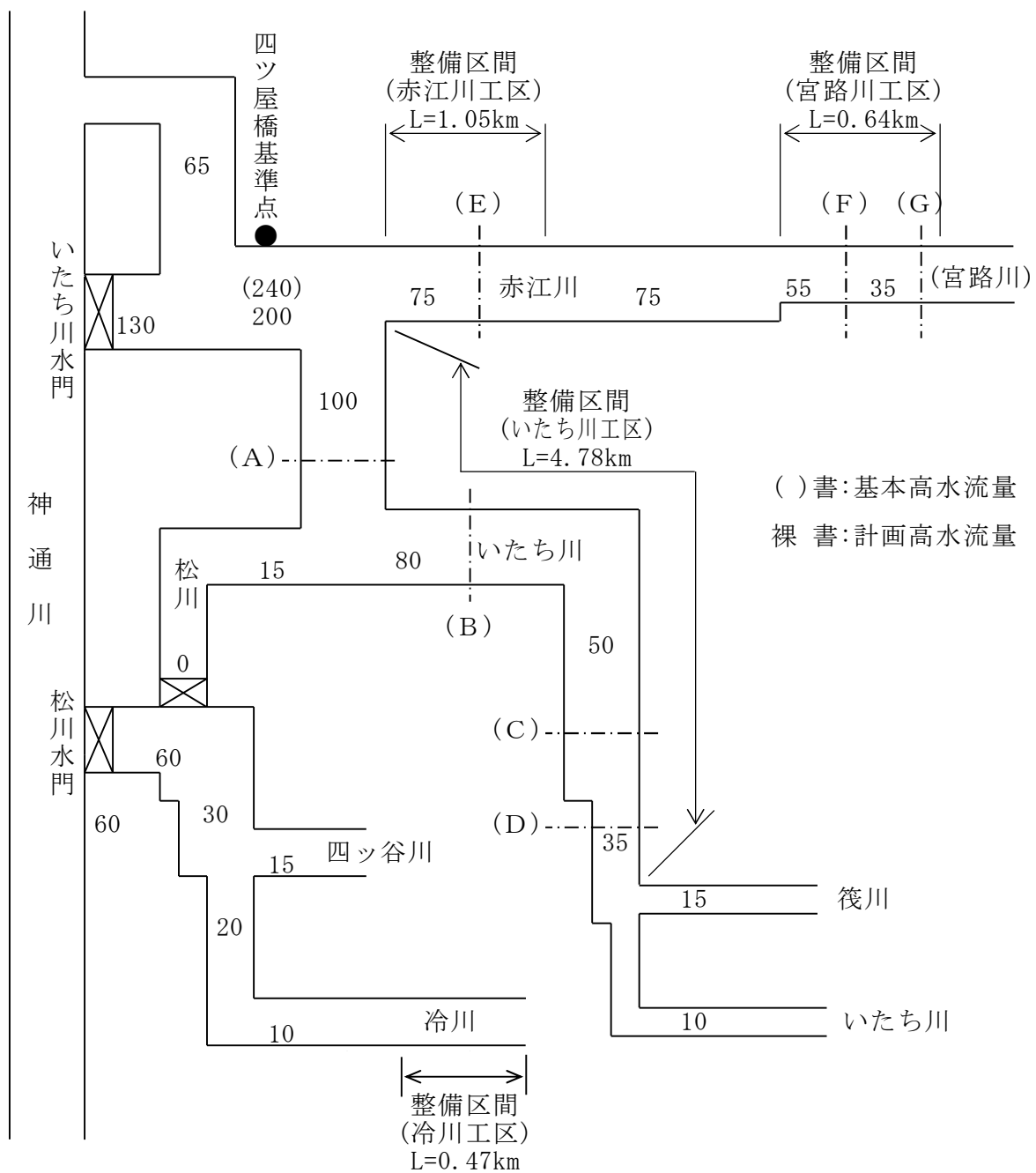
図 3 - 2 計画高水流量配分図
