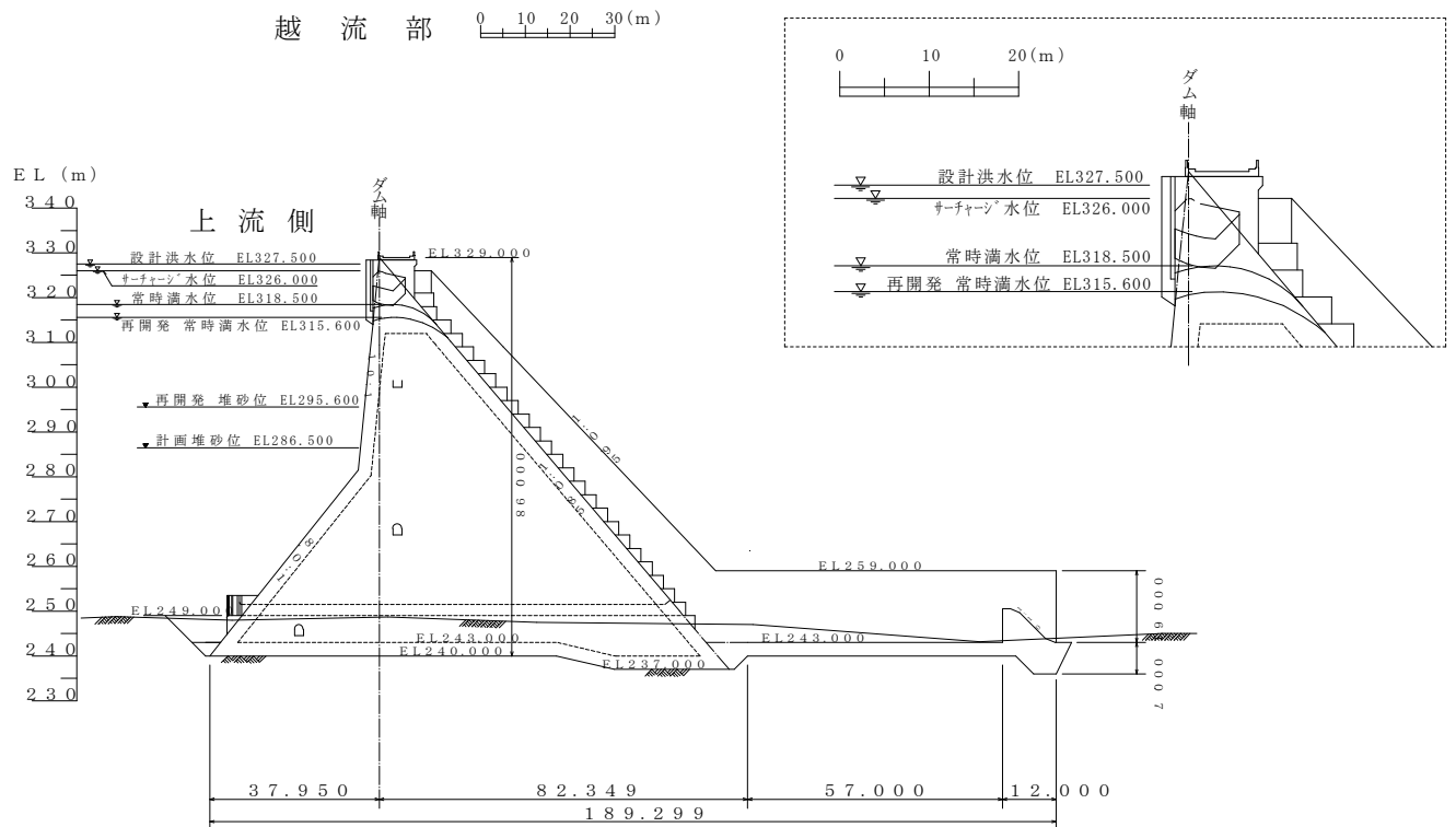
図 3 - 10 越流部標準横断面図
