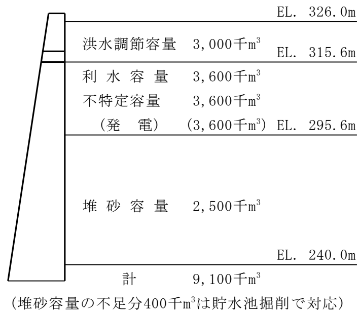
図 3 - 9 再開発後の貯水池容量配分図
