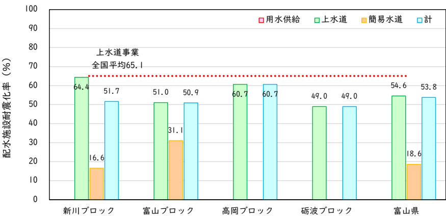
図 4-17 配水施設の耐震化率
