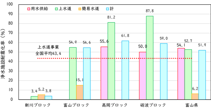
図 4-16 浄水施設の耐震化率
