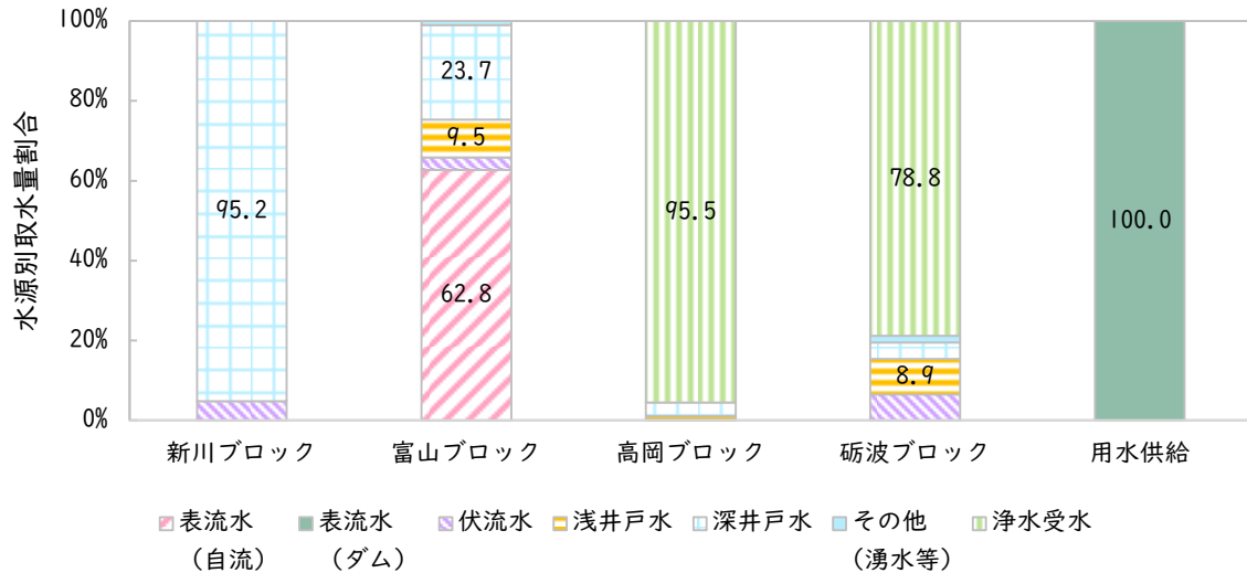
図 4-9 水源別取水割合（上水道事業及び水道用水供給事業）
