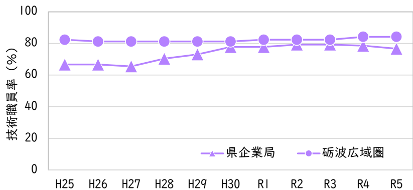
図 4-30 水道用水供給事業における技術職員率（臨時職員等を除く）
