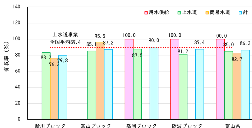
図 4-37 有収率
