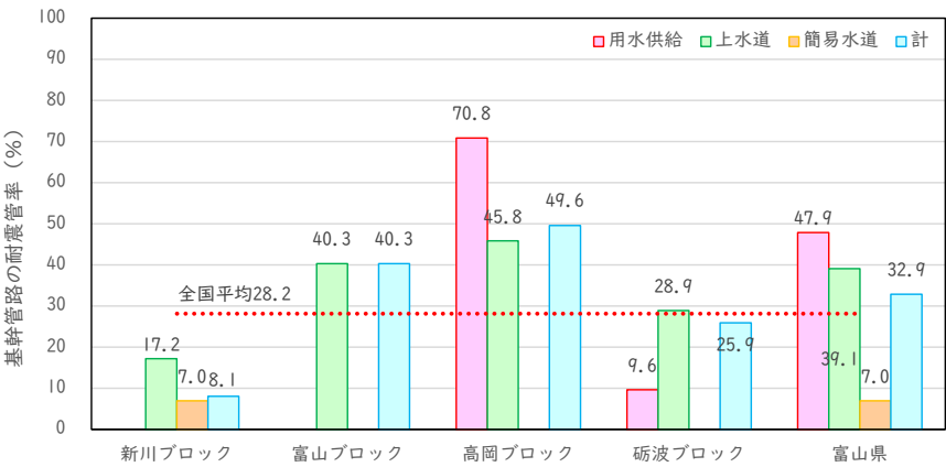
図 4-19 基幹管路の耐震管率
