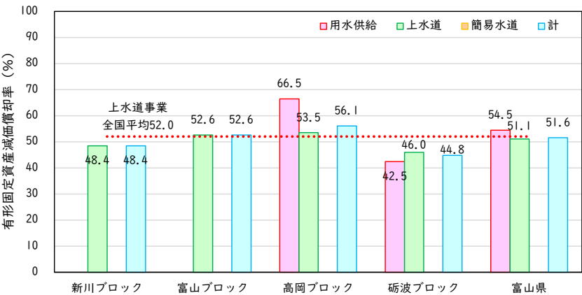
図 4-40 有形固定資産減価償却率
