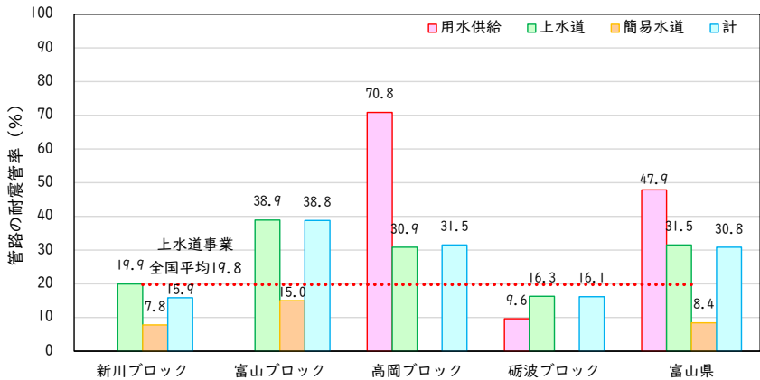
図 4-18 管路の耐震管率
