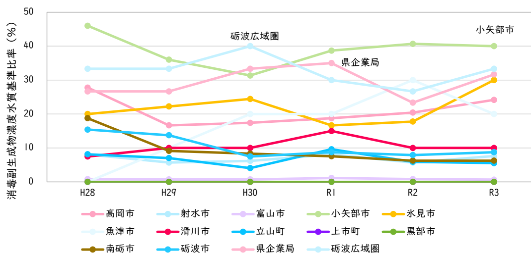
図 4-52 消毒副生成物水質基準比率 (PI)
