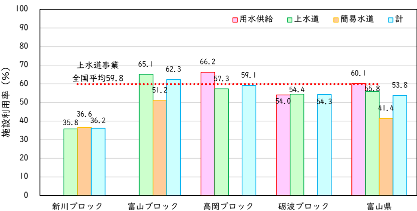
図 4-41 施設利用率
