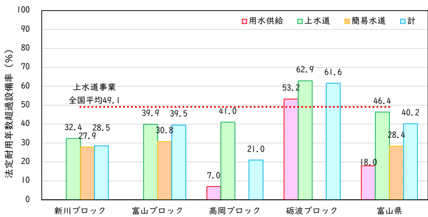
図 4-11 法定耐用年数超過設備率
