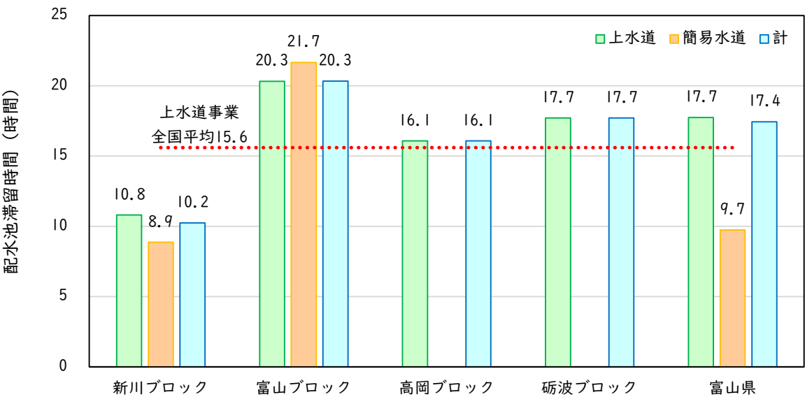
図 4-7 配水池滞留時間
