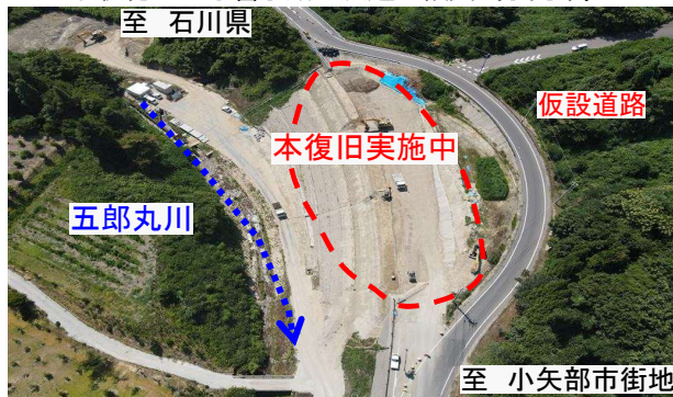
崩落した国道359号（小矢部市）
