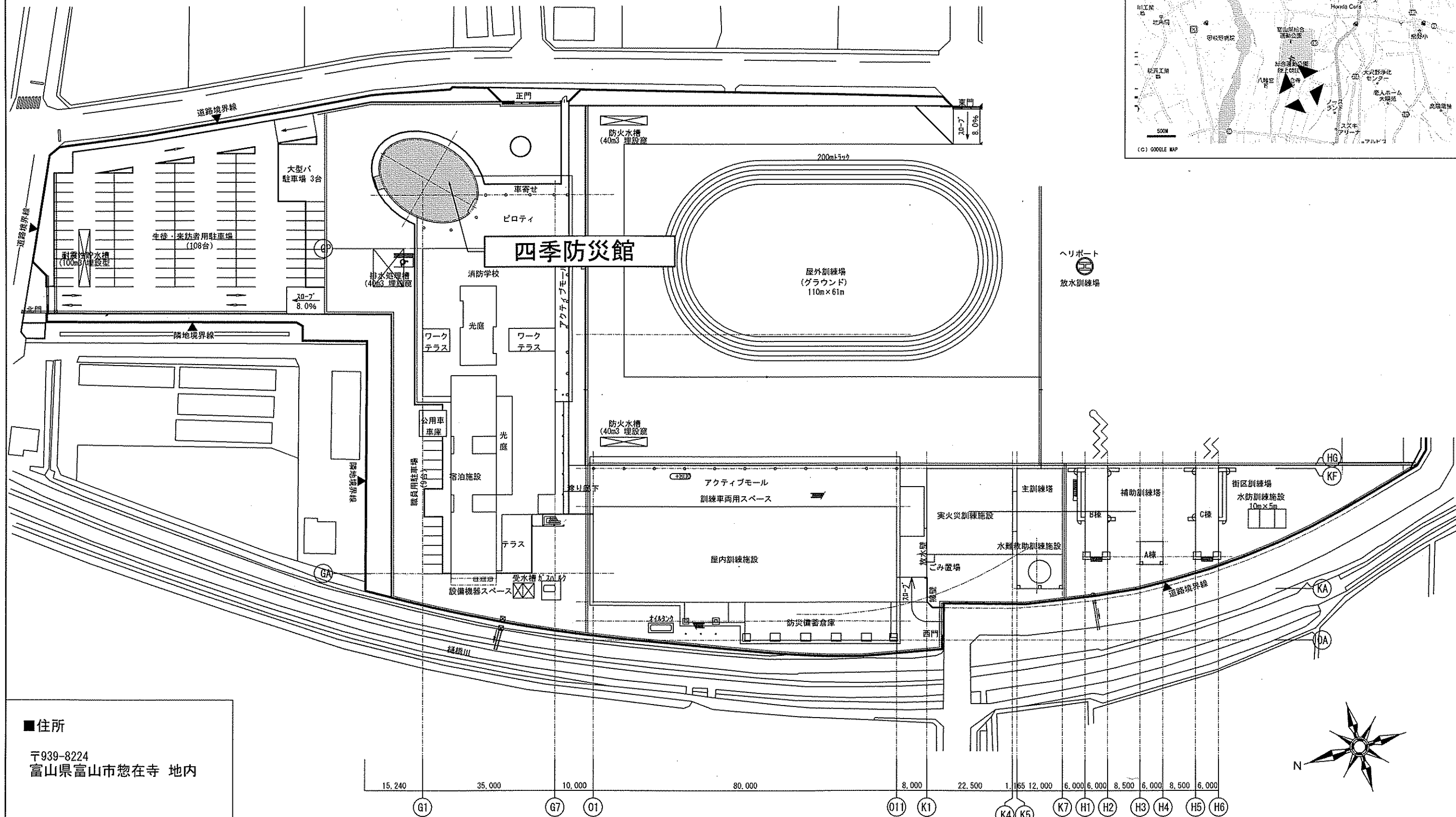
四季防災館 施設配置図
