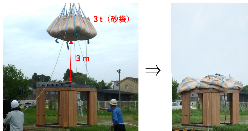
落下試験方法（6月27日の予備実験）
