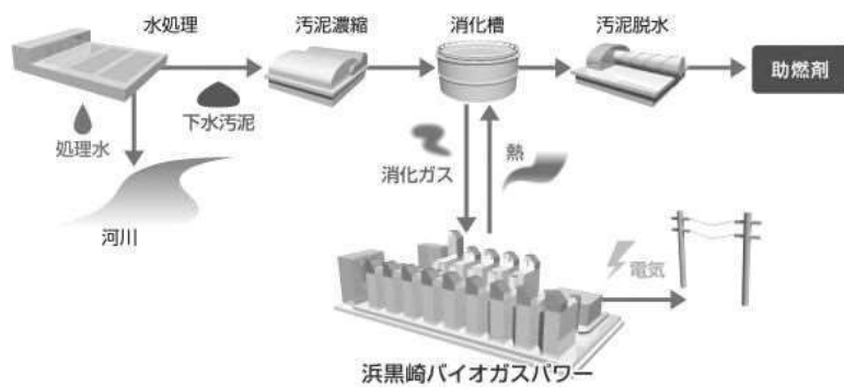
消化ガス発電施設
