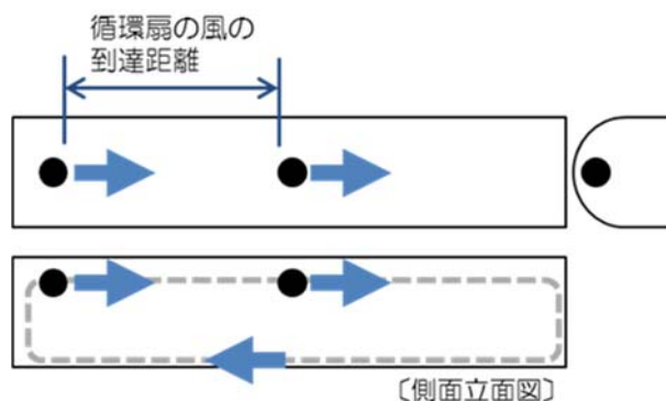
間口の狭い温室での循環扇の設置（例）
