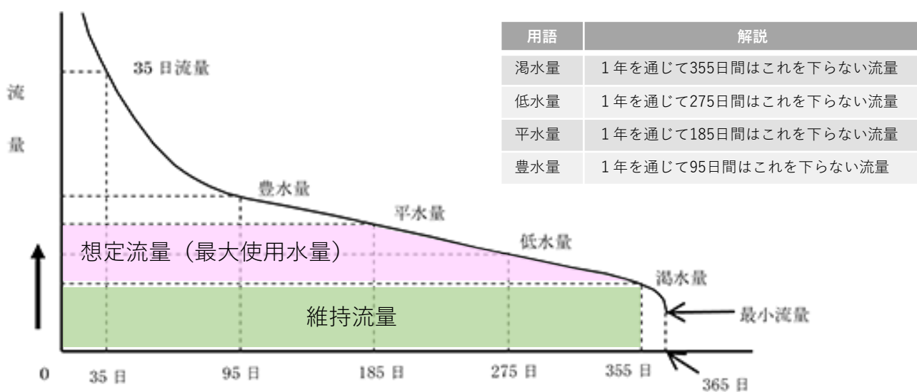
流況曲線と使用水量のイメージ
