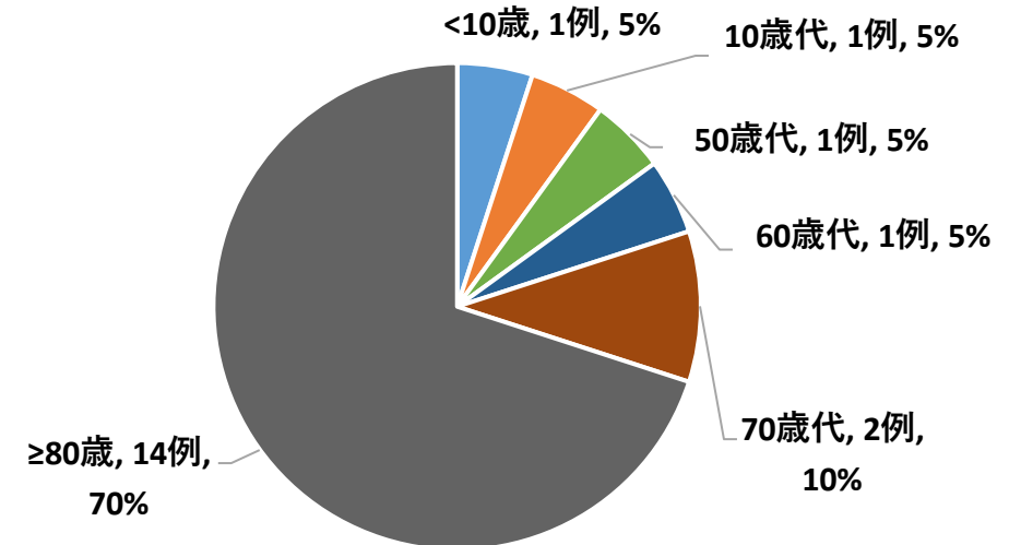
図5. COVID-19入院サーベイランス 年代分布（第10週、20例）
