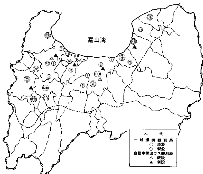
図2-6 大気汚染常時観測局の適正配置計画図
