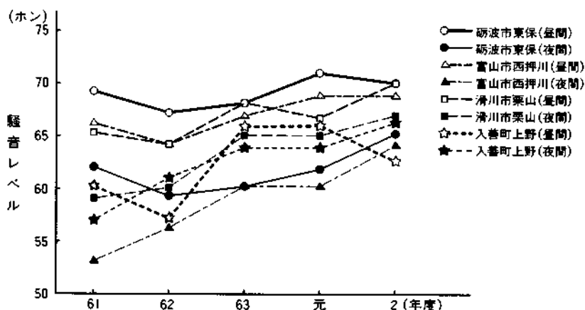
図2-19 騒音レベルの年度別推移
