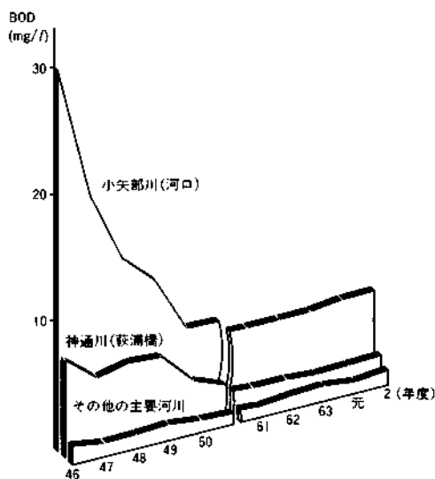
図1-6 河川及び海域の水質の推移
