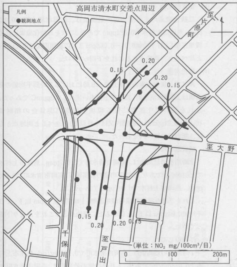
図2-8 交差点周辺における二酸化窒素濃度分布
