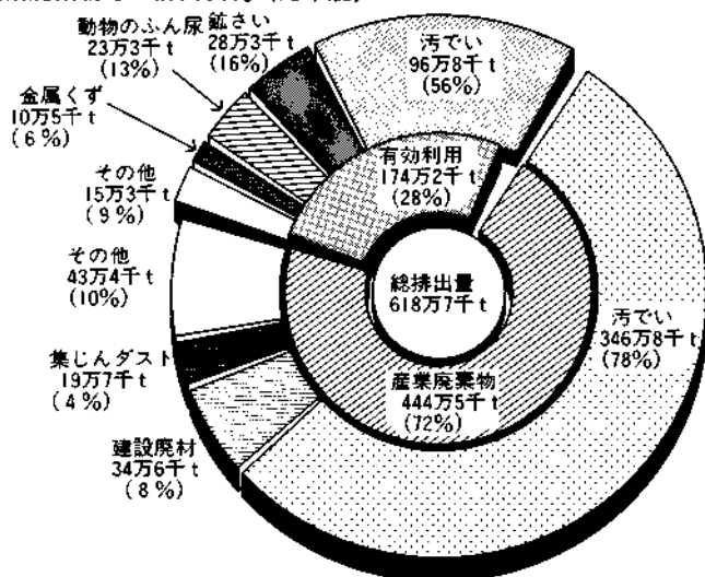
図1-22 産業廃棄物の処理状況（元年度）
