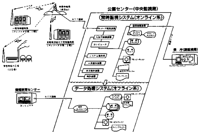
図2-5 大気汚染監視テレメータシステムの概要図
