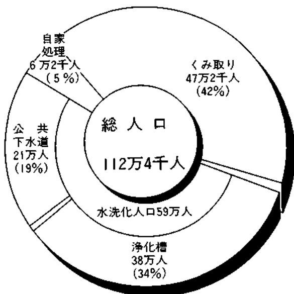
図1-19 し尿の処理状況 (元年度)
