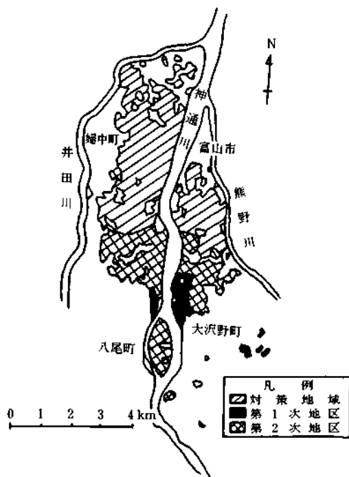
図2-21 第1次、第2次対策計画策定地域位置図
