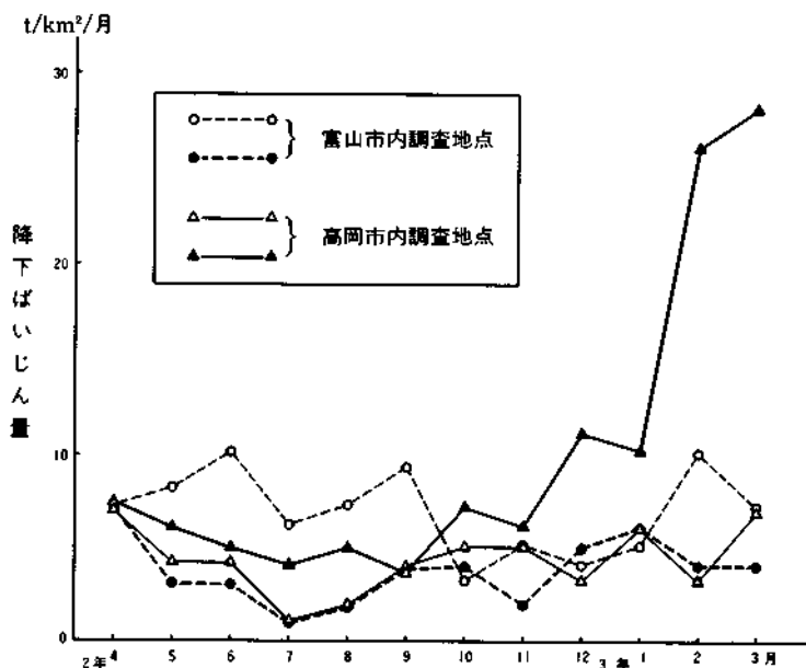
図2-9 主要測定地点における降下ばいじん量の経年変化（2年度）
