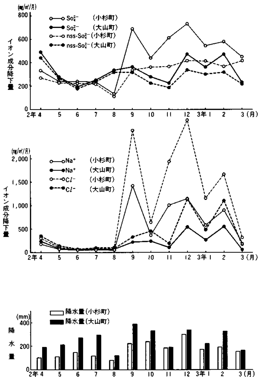
図2-11 主要イオン成分降下量、降水量の月別推移（2年度）
