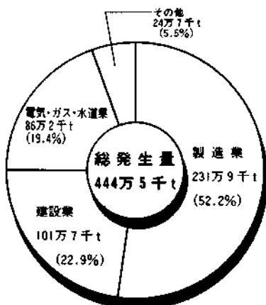
図2-26 業種別発生量（元年度）
