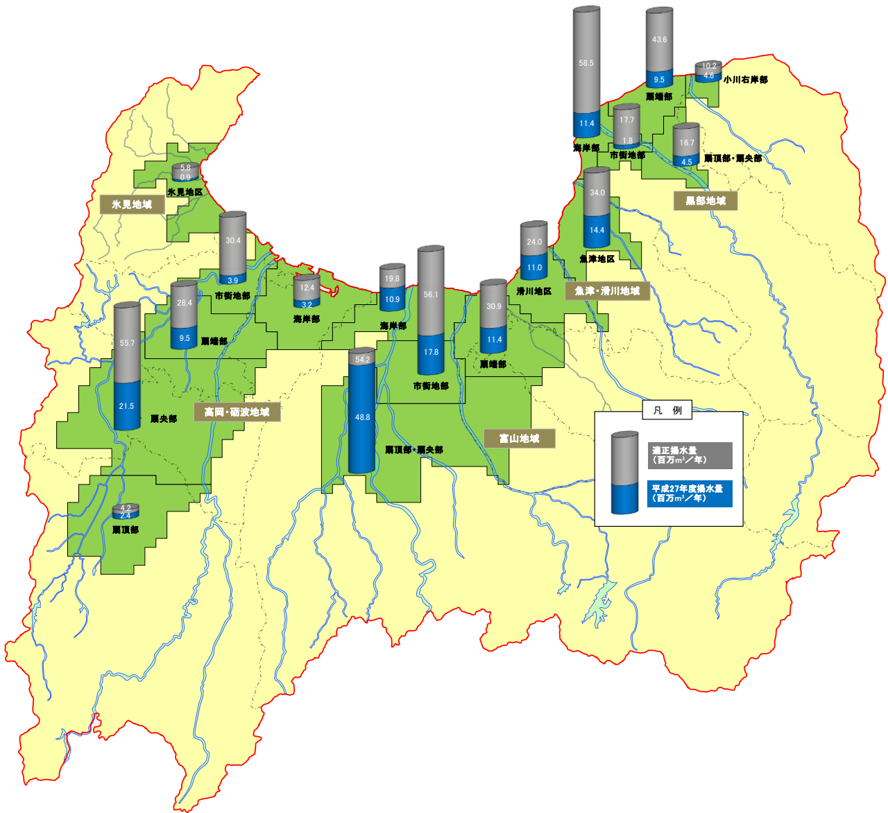
図1 平成27年度地下水揚水量と適正揚水量
