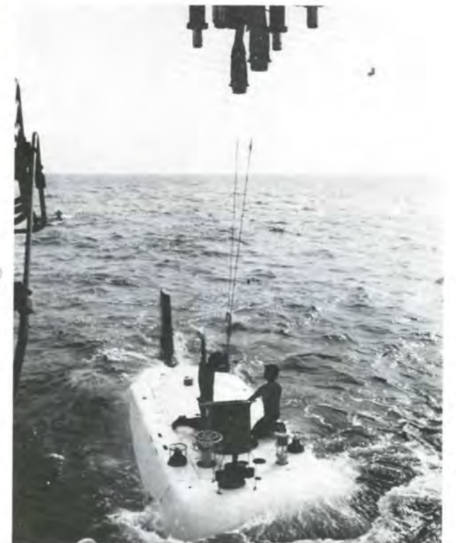
富山湾の調査を終え浮上した「しんかい2000」を引きあげる
