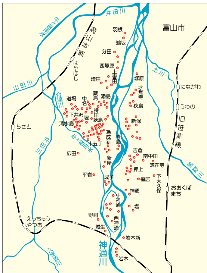
イタイイタイ病患者発生地域図 (イタイイタイ病第1合同研究会(1963(昭和38)年6月)資料の図表より作成)
