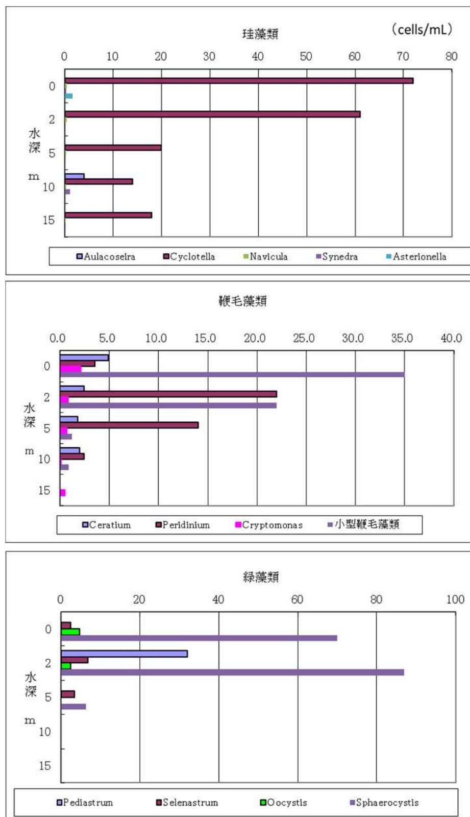
図-6 子撫川ダム湖の植物プランクトンの垂直分布（8月）
