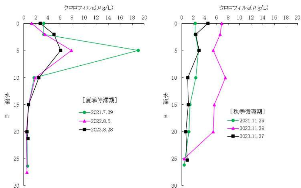
図－3 子撫川ダム湖のクロロフィル a
