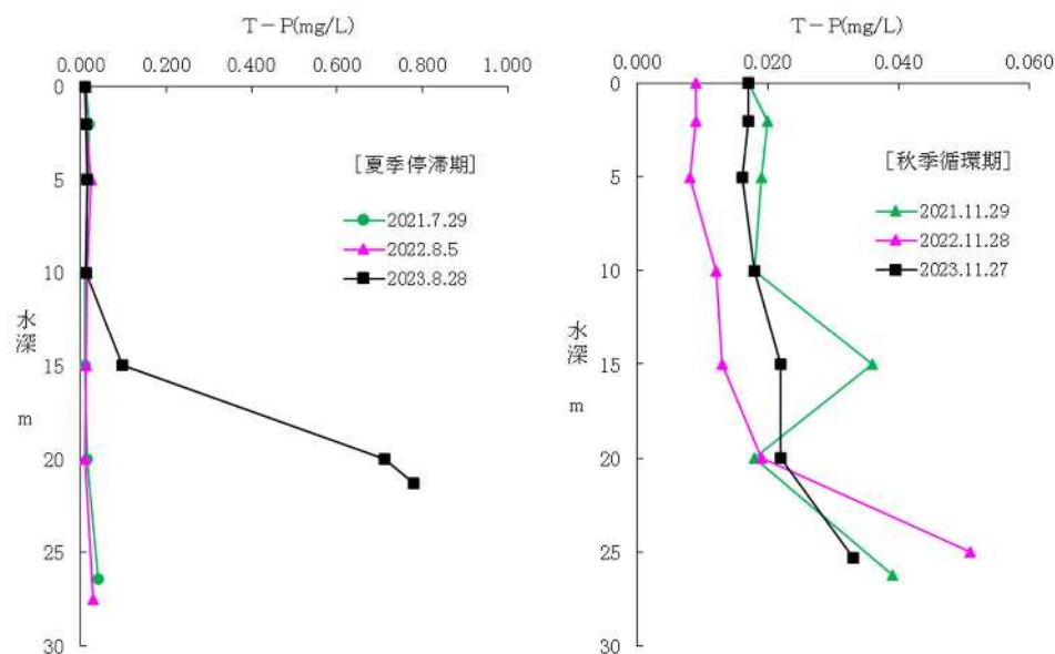
図－５ 子撫川ダム湖の T-P
