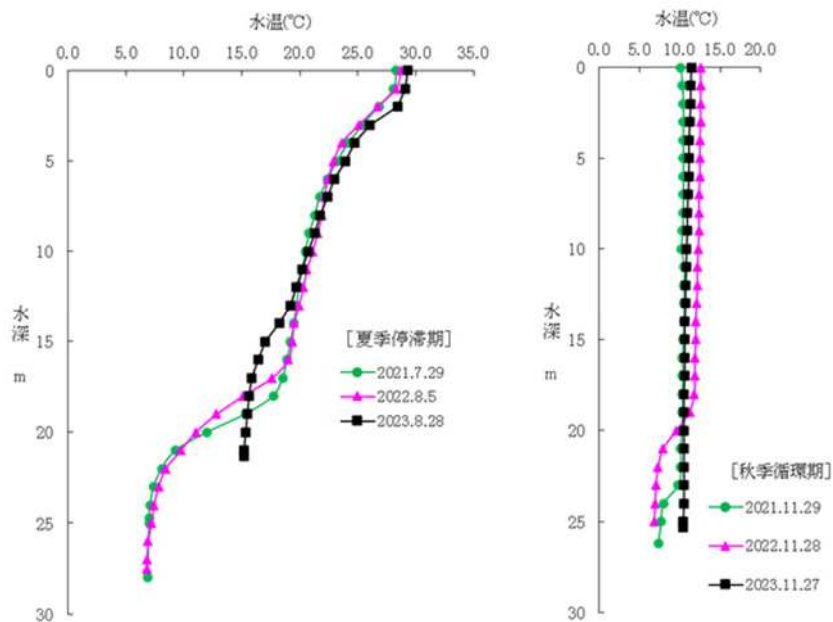
図－２ 子撫川ダム湖の水温鉛直分布
