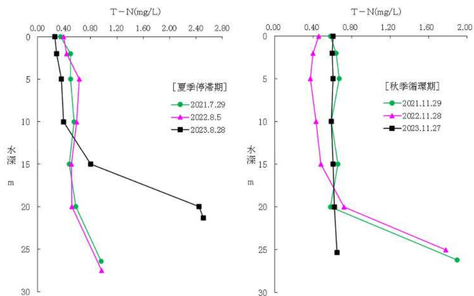
図－4 子撫川ダム湖の T-N
