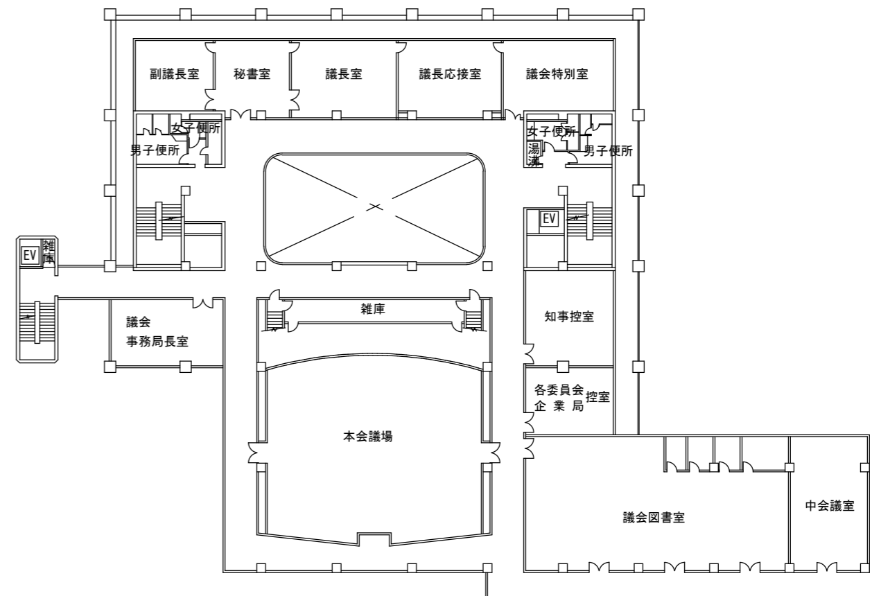
3階平面図
