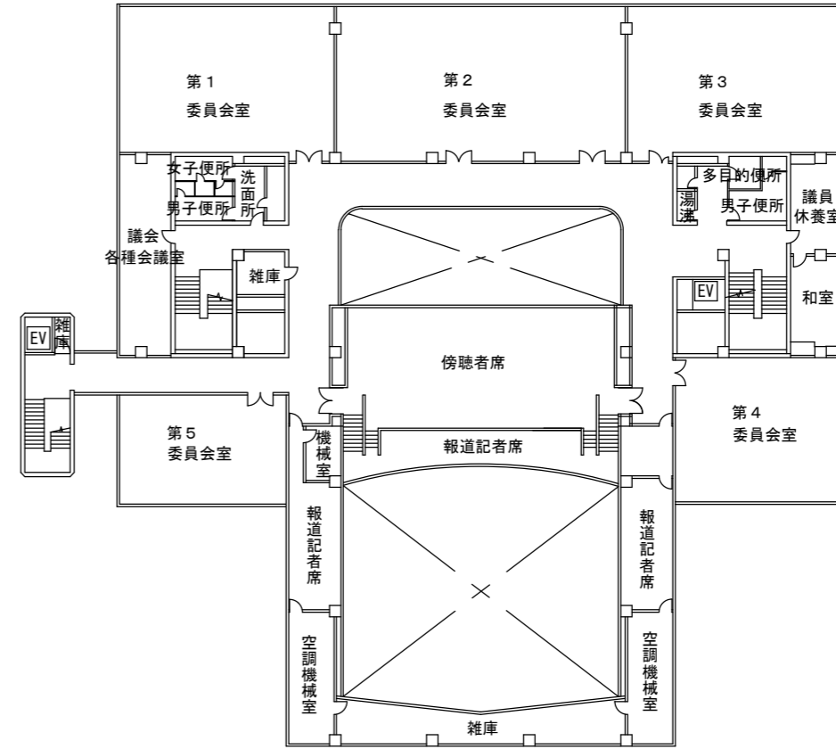
4階平面図
