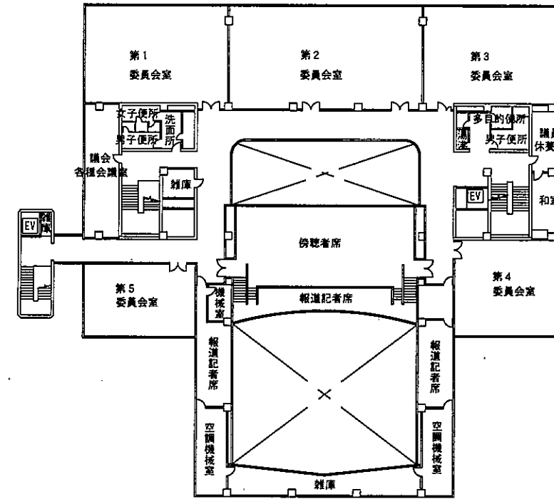
4階平面図
