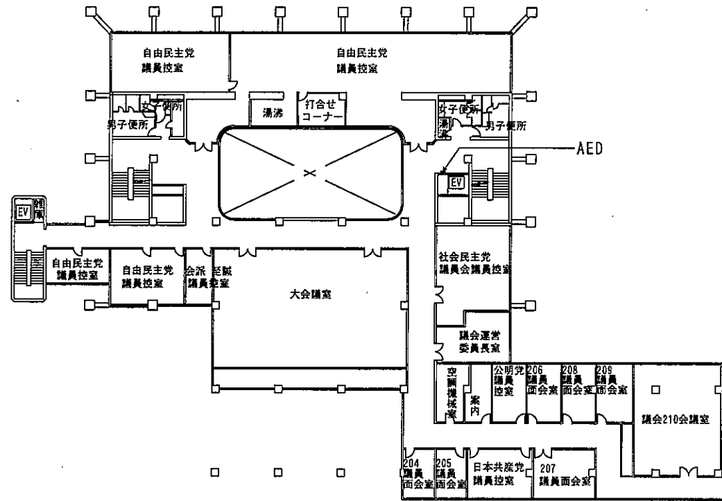
2階平面図
