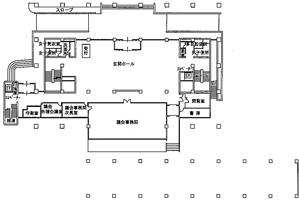
1階平面図
