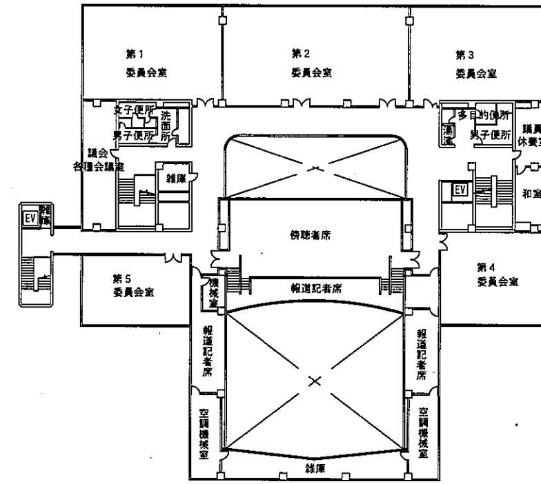
4階平面図
