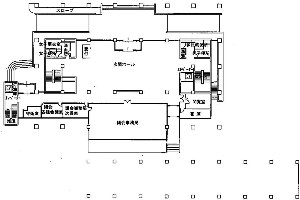
1階平面図
