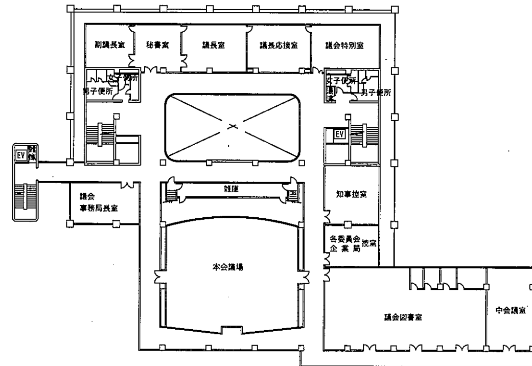
3階平面図
