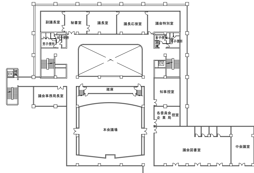
3階平面図
