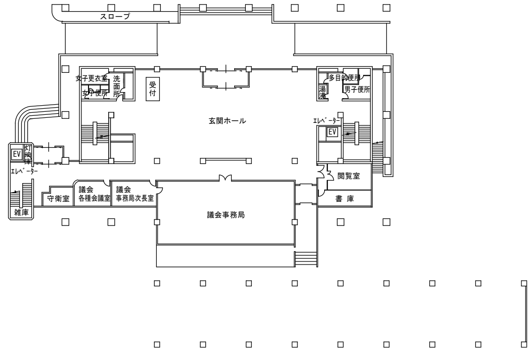
1階平面図
