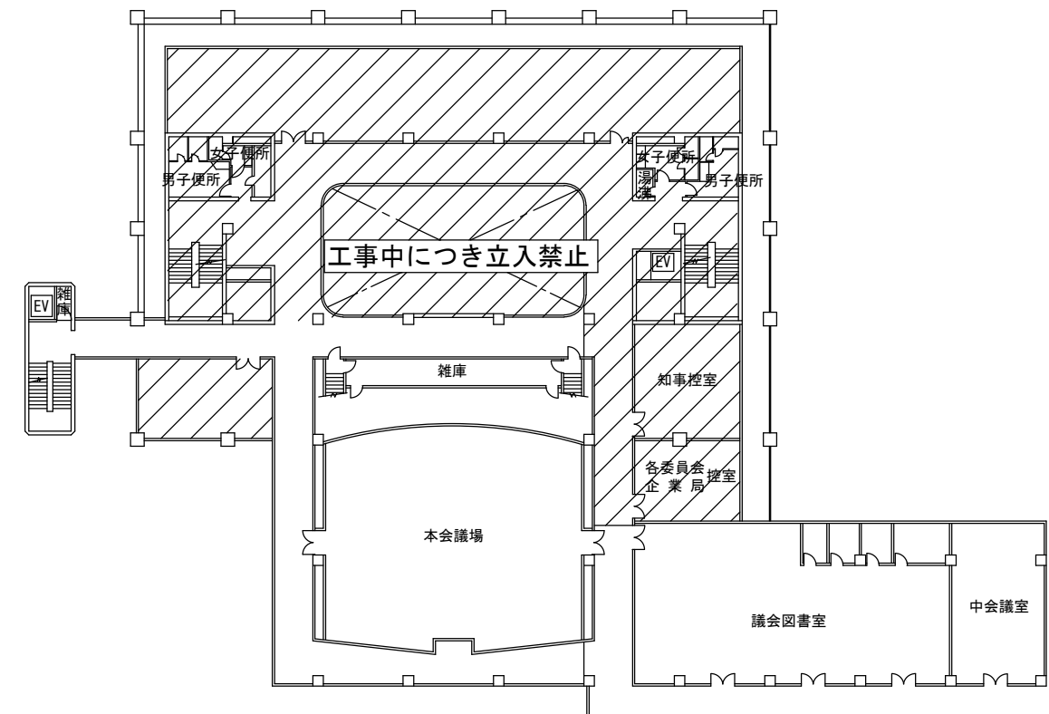
3階平面図
