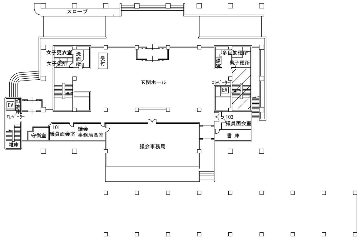
1階平面図
