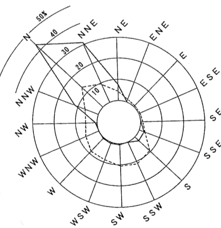
風向風速図
