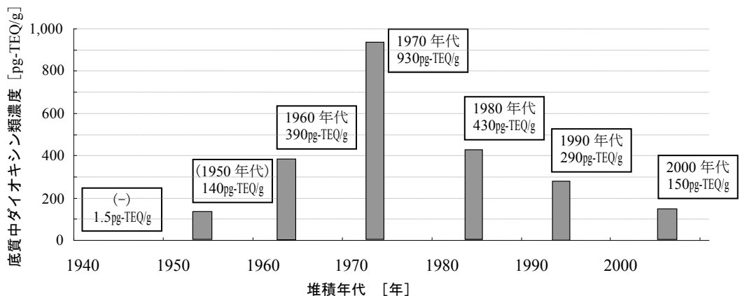
図 14 ダイオキシン類の堆積状況の推移（住友運河）
