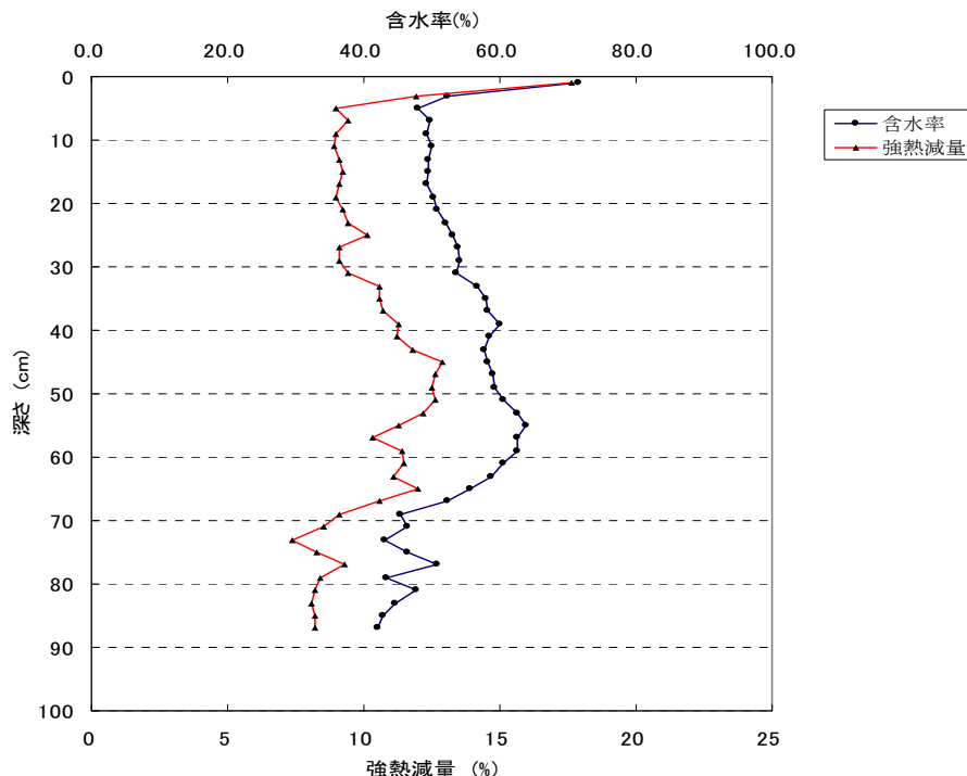
図 6 含水率及び強熱減量の分析結果（富岩運河）
