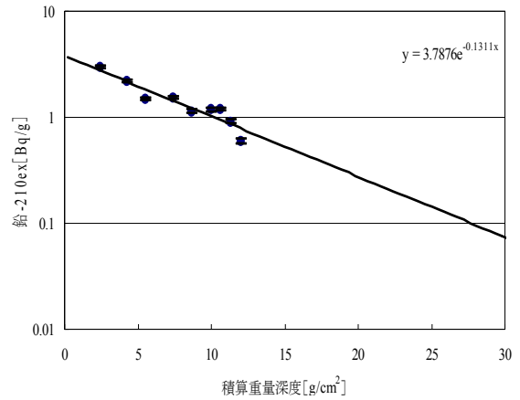
図 11 積算重量深度と鉛-210ex との関係（住友運河）
