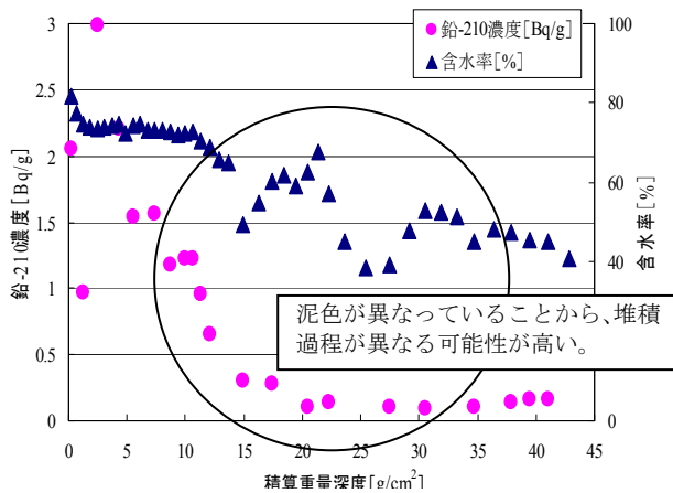
図 10 積算重量深度に対する含水率と鉛-210の結果（住友運河）
