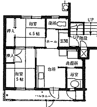
東新庄3号棟 Bタイプ (1階)
