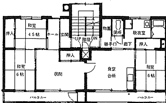
東新庄3号棟 Aタイプ (2, 3, 4階)
