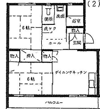
五福2号棟 Bタイプ 身障者向住宅
