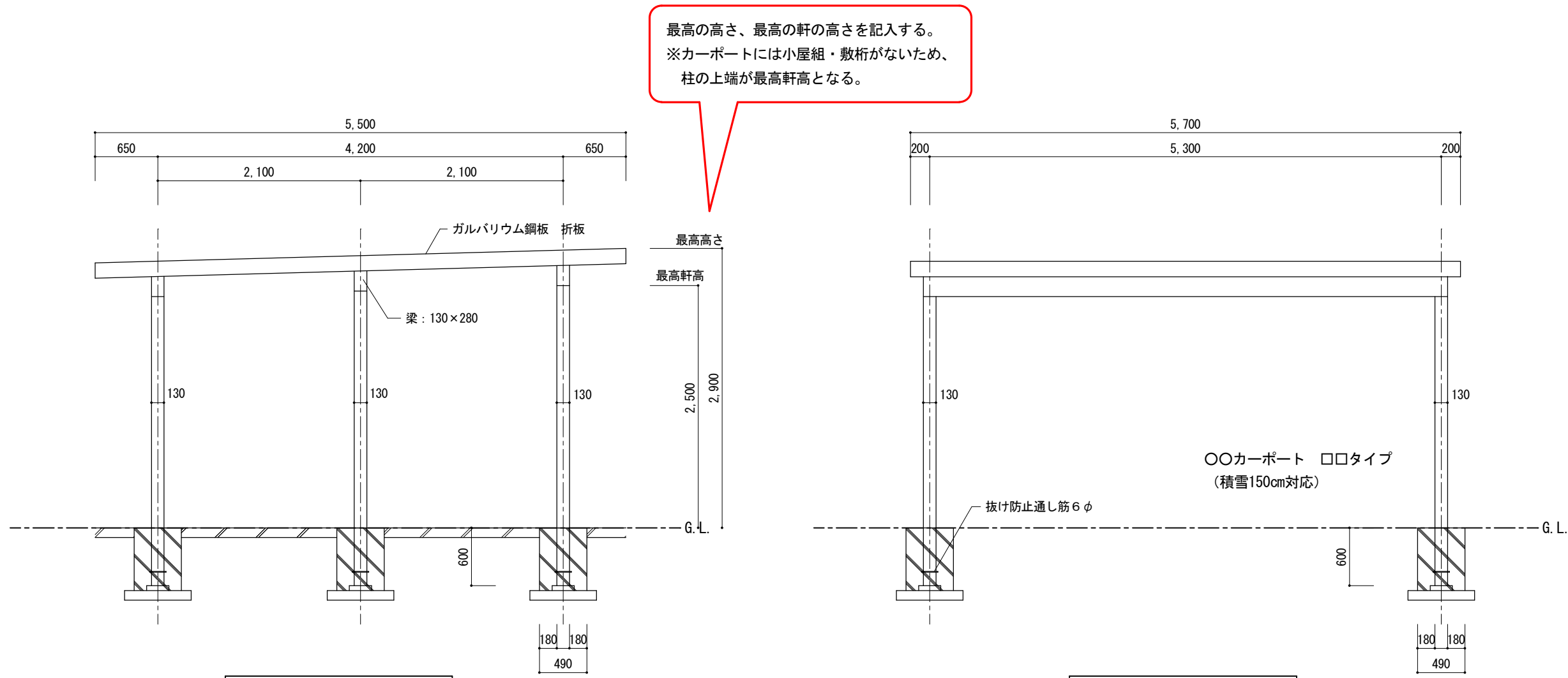
東側立面図 1/100
