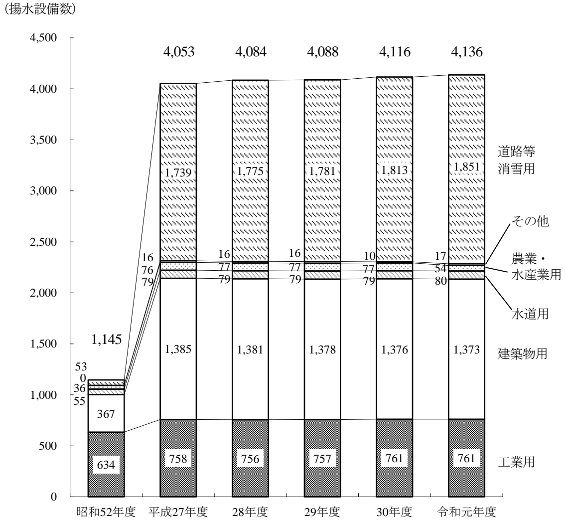
図2 揚水設備数の推移
